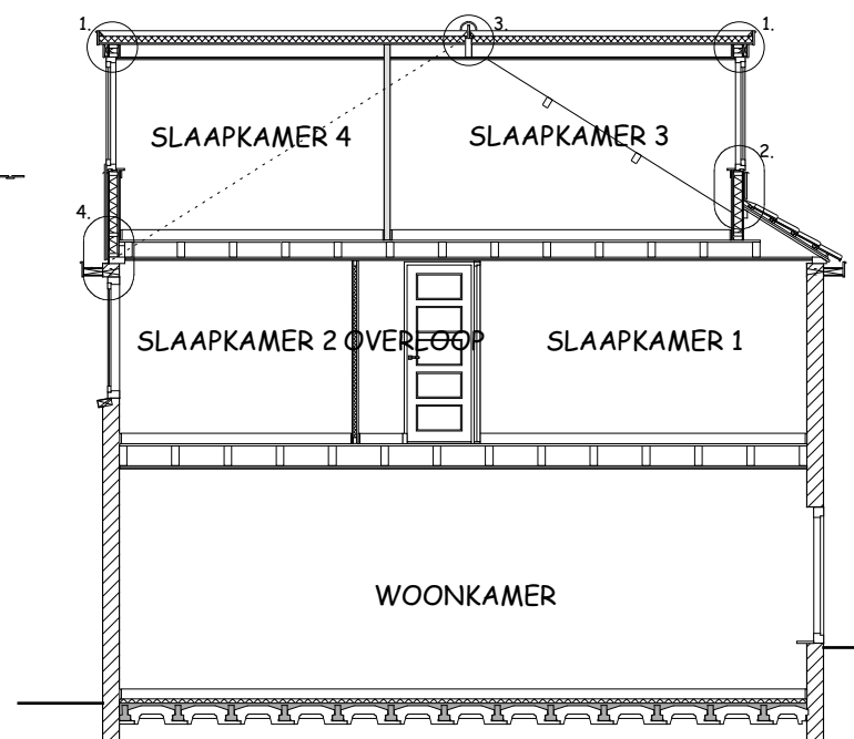
LANGSDOORSNEDE NIEUW
