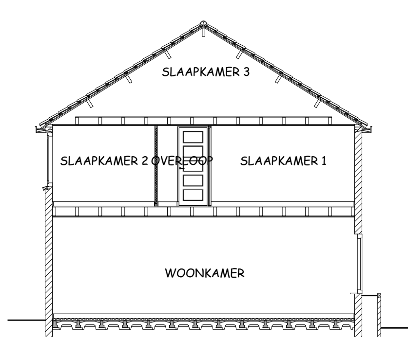
LANGSDOORSNEDE BESTAAND
