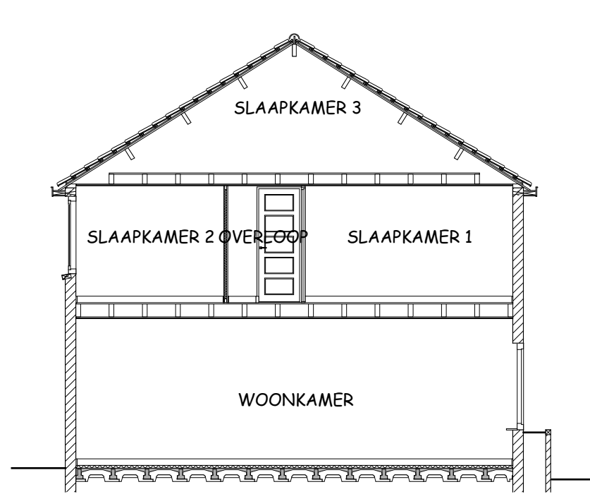
LANGSDOORSNEDE BESTAAND
