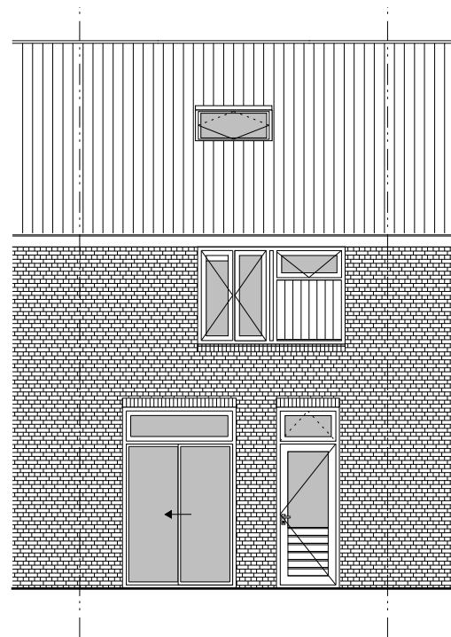
ACHTERGEVEL BESTAAND
